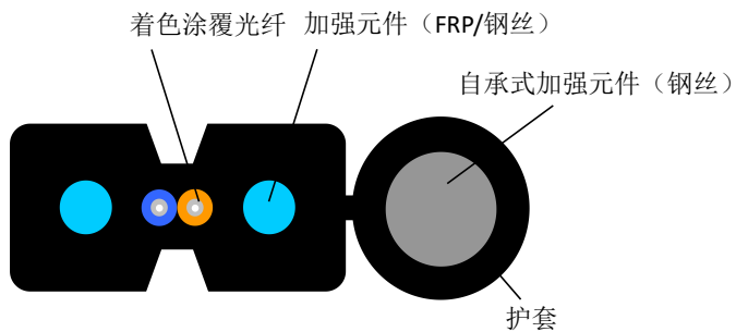
自承式蝶形引入光缆 I 型
